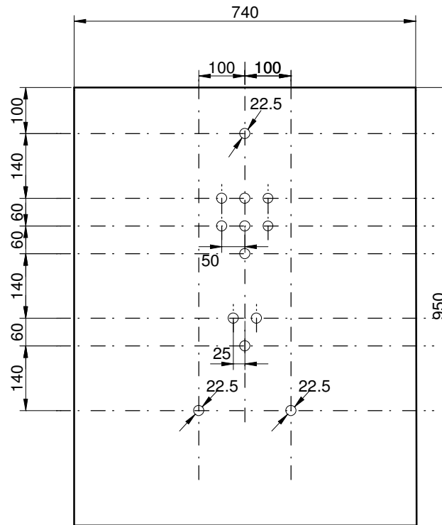
PLAN DE DECOUPE PORTE INTERIEURE
