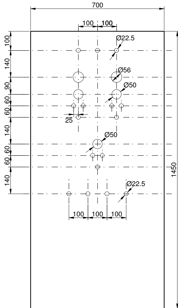
PLAN DE DECOUPE PORTE INTERIEURE
