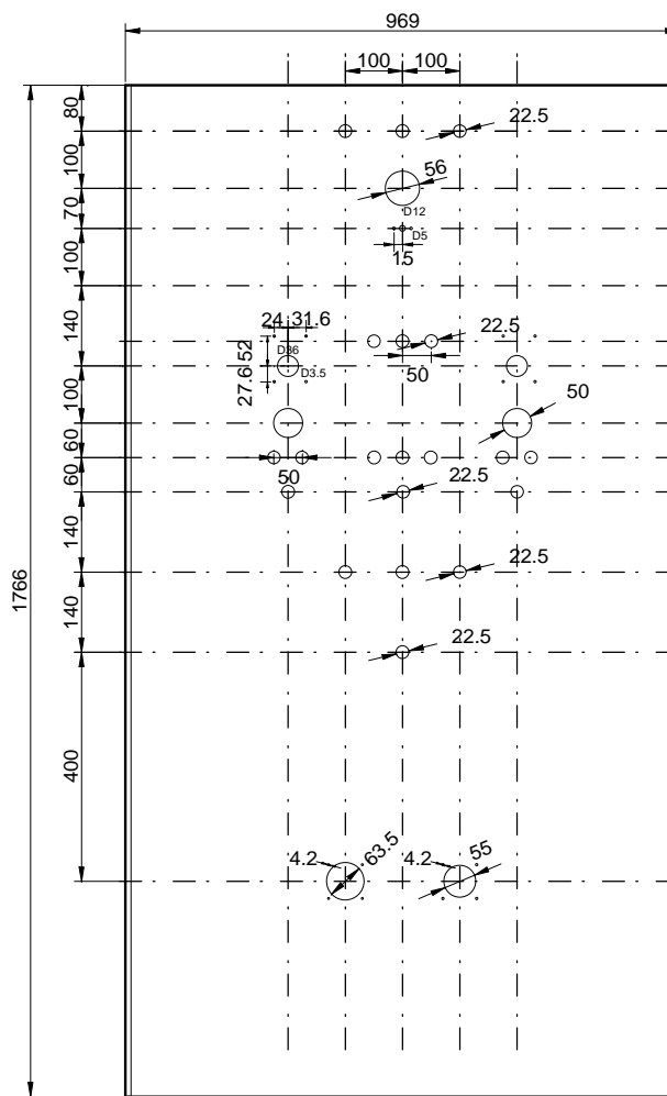
PLAN DE DECOUPE
