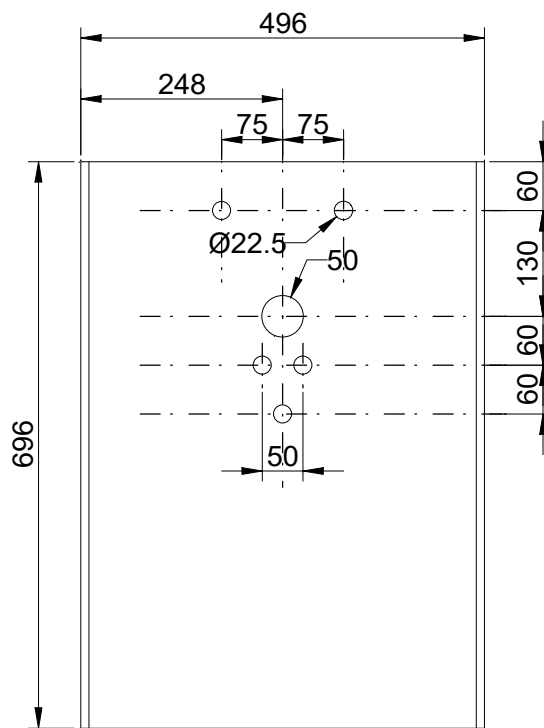
PLAN DE DECOUPE
