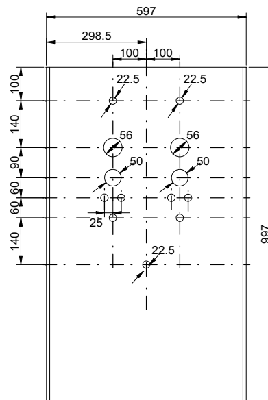
PLAN DE DECOUPE PORTE INTERIEURE
