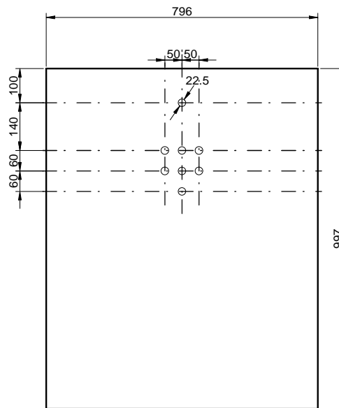
PLAN DE DECOUPE PORTE INTERIEURE
