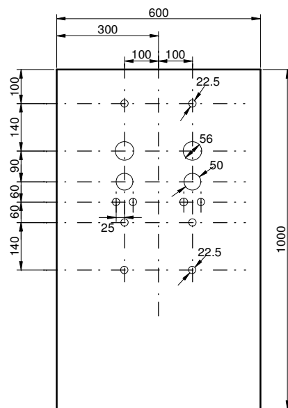
PLAN DE DECOUPE PORTE INTERIEURE
