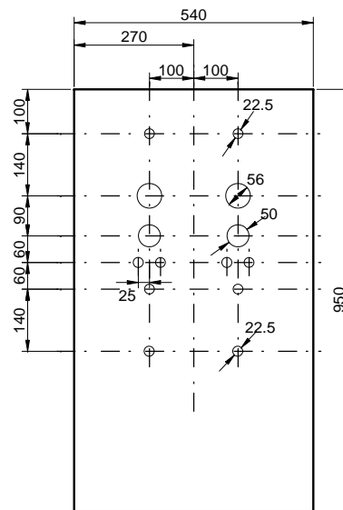
PLAN DE DECOUPE PORTE INTERIEURE
