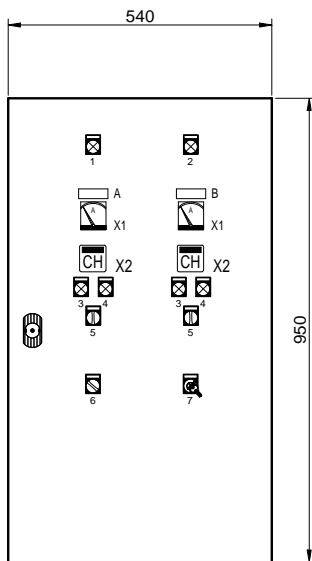
PORTE INTERIEURE
