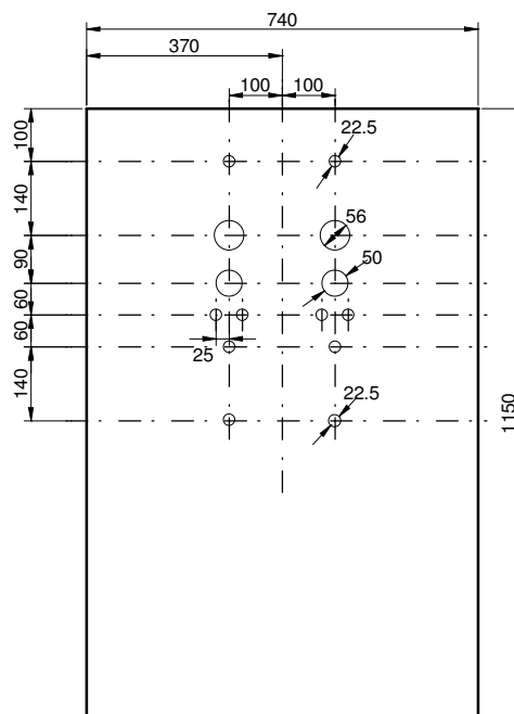
PLAN DE DECOUPE PORTE INTERIEURE
