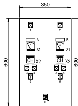
IMPLANTATION PLATINE INTERIEURE
