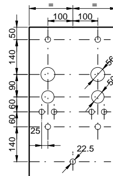
PLAN DE DECOUPE PLATINE INTERIEURE
