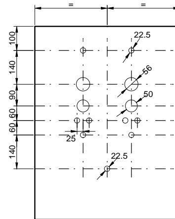
PLAN DE DECOUPE
