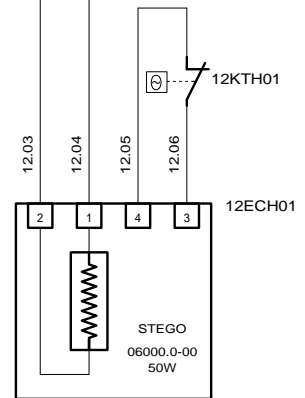
CHAUFFAGE ARMOIRE
