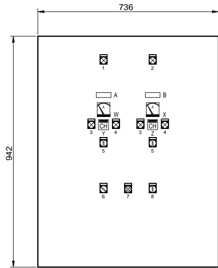
PORTE INTERNE (dimensions utiles : 800x640mm)
