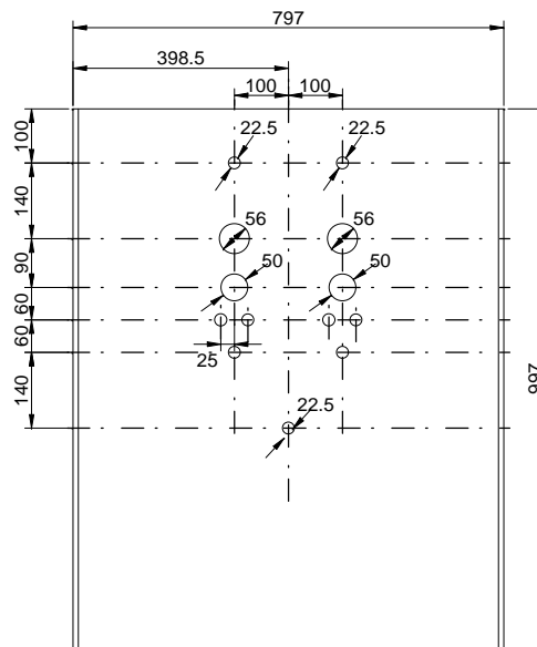
PLAN DE COUPE PORTE INTERIEURE
