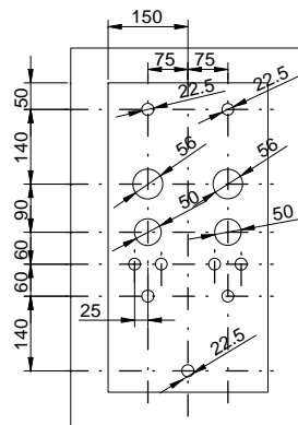
PLATINE INTERIEURE
