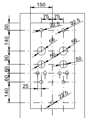
PLATINE INTERIEURE
