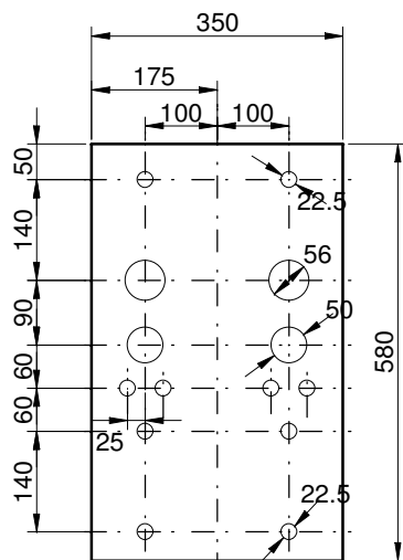
PLAN DE DECOUPE PLATINE INTERIEURE
