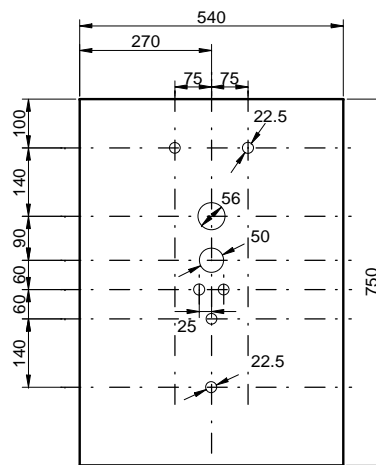
PLAN DE DECOUPE PORTE INTERIEURE
