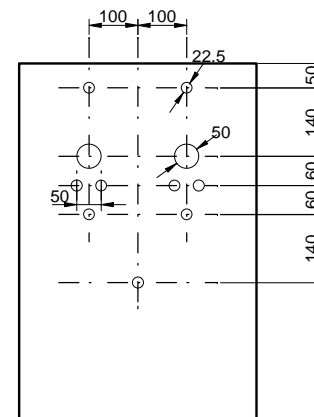
PLAN DE DECOUPE PORTE INTERIEURE
