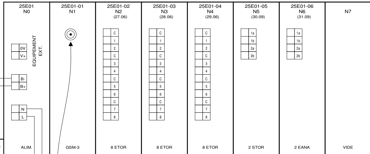
SOFREL S550 (VUE DE DESSOUS)
