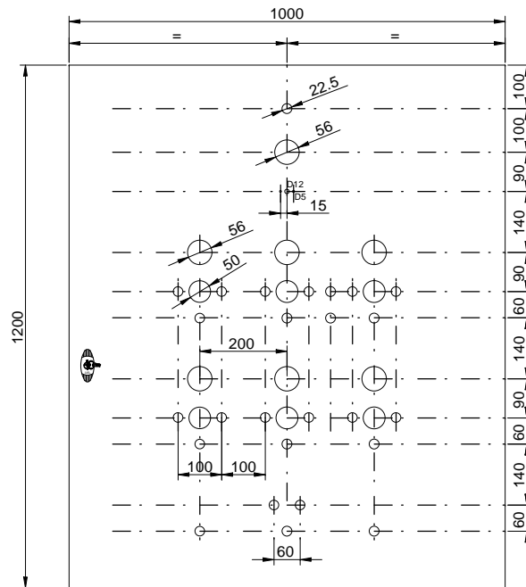
PLAN DE DECOUPE
